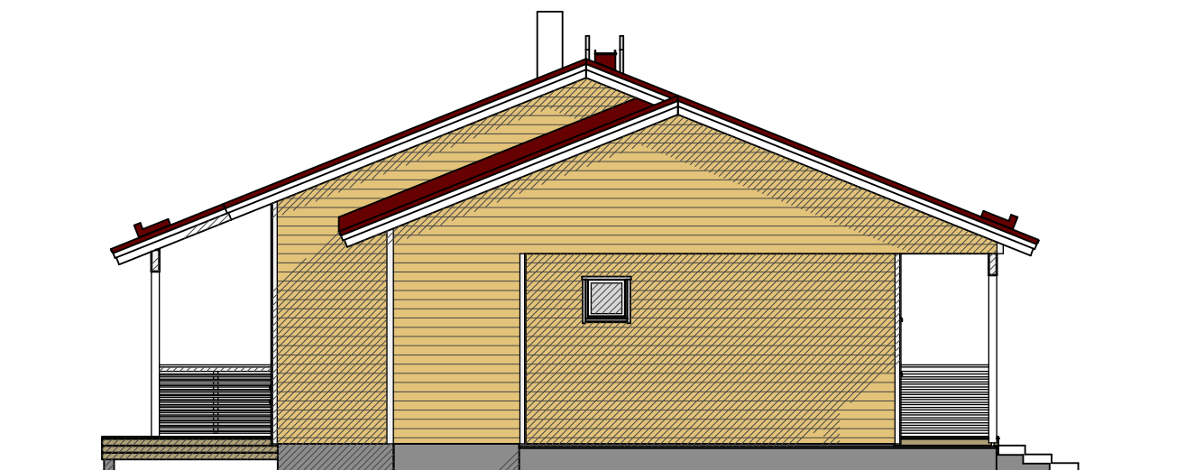
JULKISIVU VASEMMALTA
